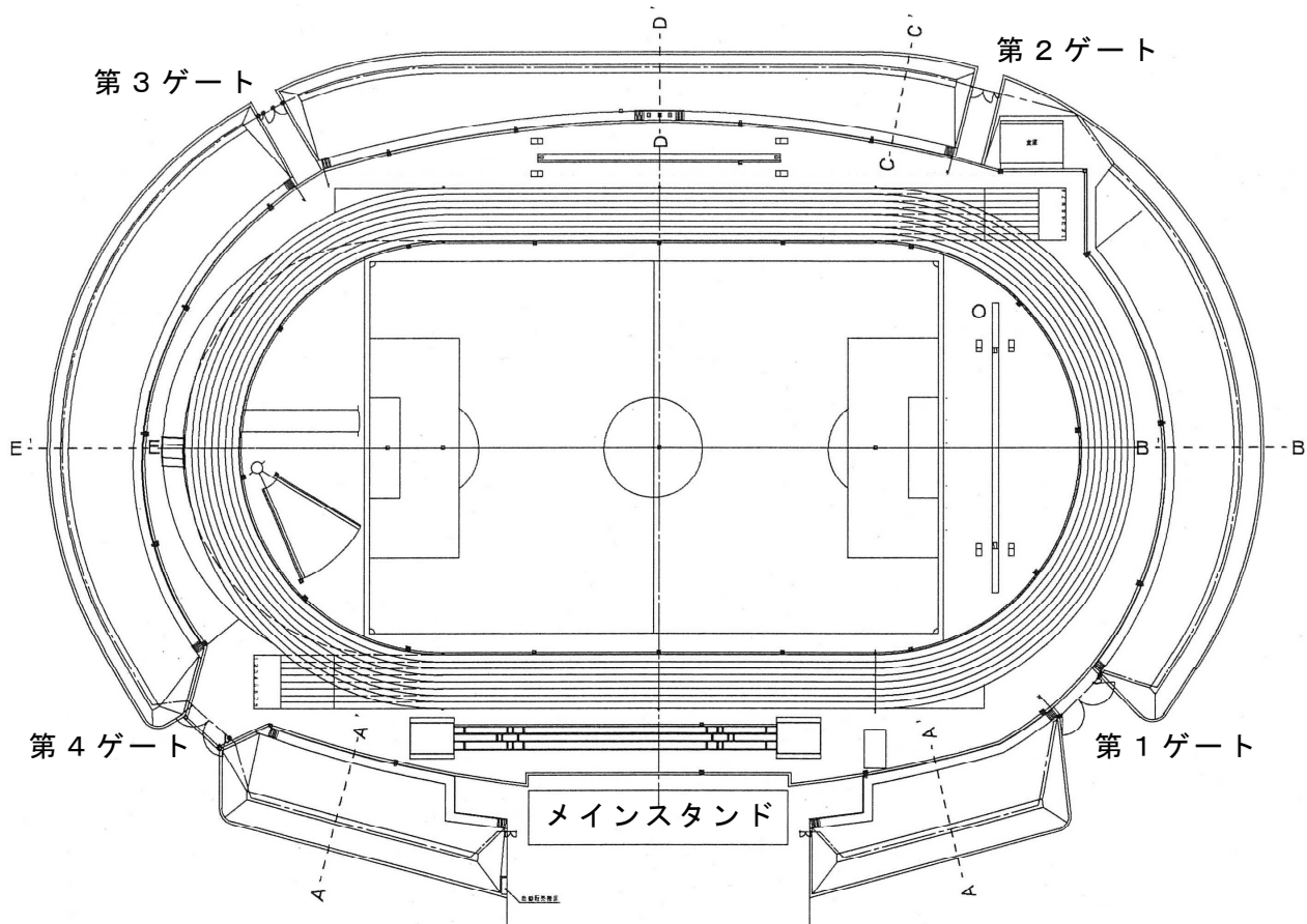
競技場平面図 S=1:1000
